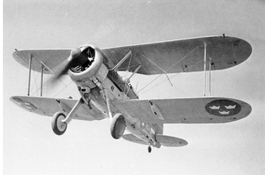
Jaktflygplan J8 Gloster Gladiator. Gloster Aircraft Company England- Inköptes 1937 Antal av 55 Operativ drift 1937-1947 Beväpning 4 st 8 mm ksp m/22F Kunde medföra 4 st 12-kilos sprängbomber för lätta attackuppdrag
