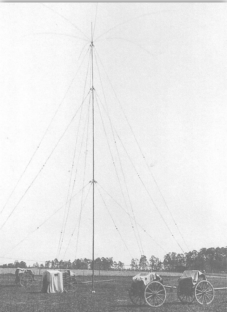
Åkande fältradiostation m/17
